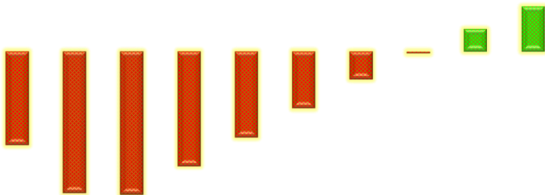
Рисунок 9.2. Динамика ЧДД
